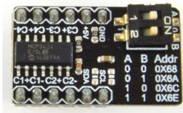
Εικόνα 12 MCP3424 DFROBOT
