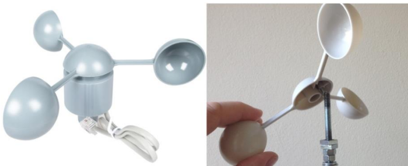
Εικόνα 13 Αισθητήρας μέτρησης ταχύτητας ανέμου SparkFun
